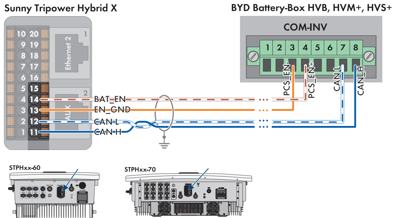
Abbildung 4: Verkabelungsprinzip für die Verschaltung von Sunny Tripower Hybrid X mit BYD Battery-Box HVB, HVM+ und HVS+.
