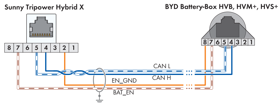
Abbildung 5: Verkabelungsprinzip: Sunny Tripower Hybrid X mit BYD Battery-Box HVB, HVM+ und HVS+.
