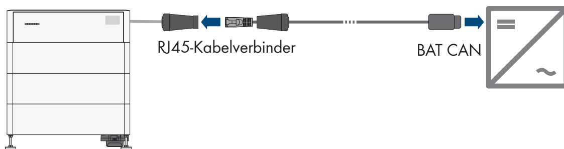
Abbildung 2: Verkabelungsprinzip mit Standard-Patchkabel Sunny Tripower Hybrid X mit SMA Storage M
