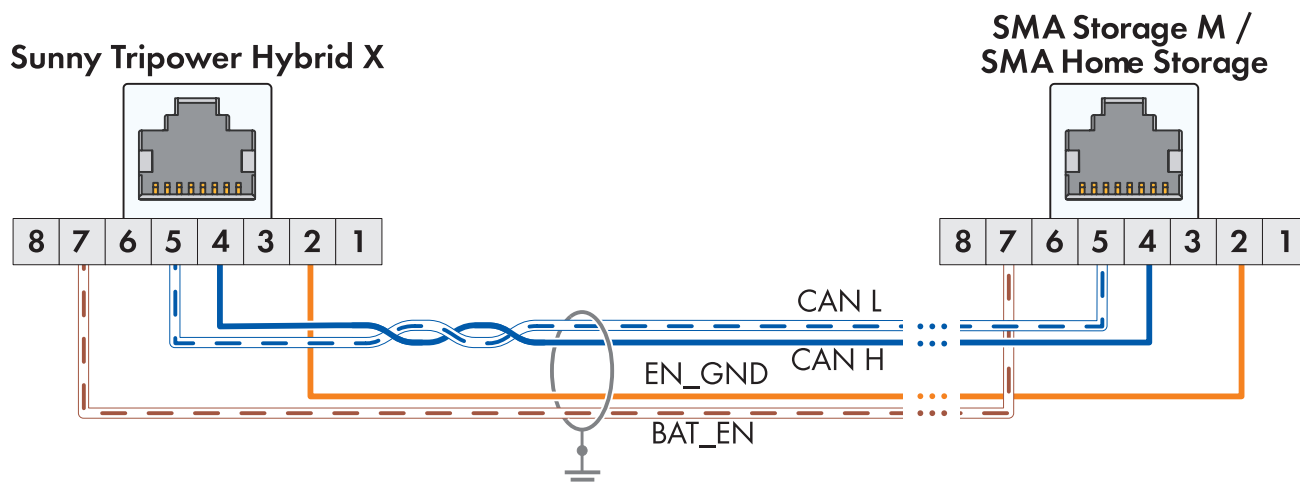
Abbildung 3: Verkabelungsprinzip Sunny Tripower Hybrid X mit SMA Home Storage und Storage M über BAT CAN (RJ45)
