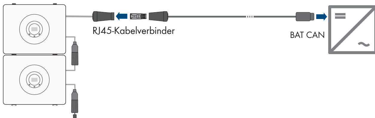
Abbildung 1: Verkabelungsprinzip mit Standard-Patchkabel Sunny Tripower Hybrid X mit SMA Home Storage
